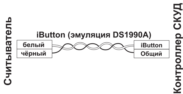
Рис. 4 Схема подключения
