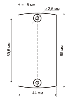
Рис.2 Габаритные размеры
