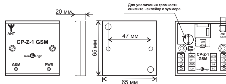
Рис.1 Габариты изделия.
