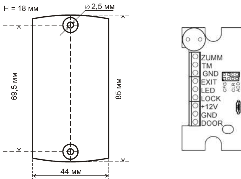
Рис.1 Габаритные размеры и расположение клемм
